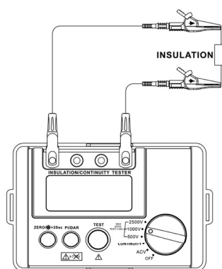
Рис. 5. Измерение сопротивления изоляции
